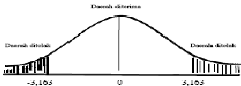
Gambar 1 Grafik Kriteria Pengujian Hipotesis
