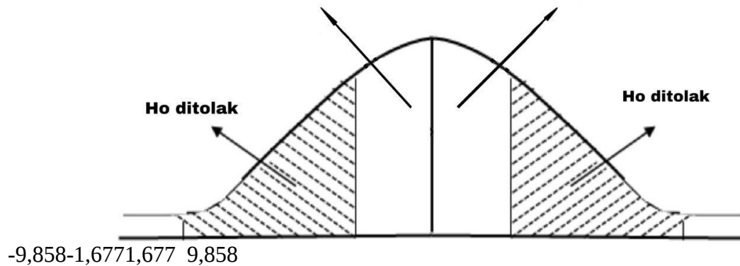
sumber: hasil diolah penulis Gambar 2 Kurva Hasil Uji Parsial (Uji t)
