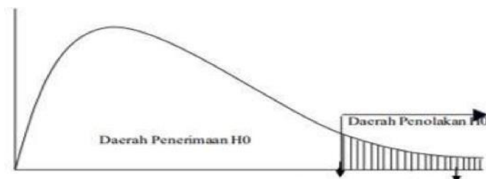
Gambar 3 Kurva Hasil Uji Simultan (Uji F)
